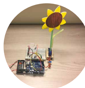
Projet d'initiation à l'électronique (impliquant moteur et programmation) faisant tourner un faux tournesol en fonction du soleil
